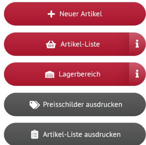
Bild 6: Artikelliste/Preisschild drucken
